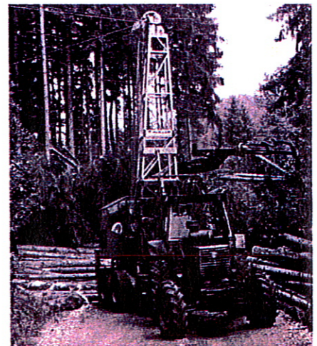
Mit einem Koller K300, aufgebaut auf einem Forwarder-Chassis, wurde die Seilbringung vorgeführt
